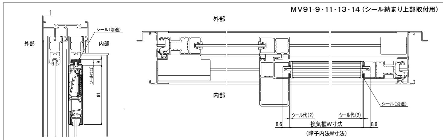
商品図
