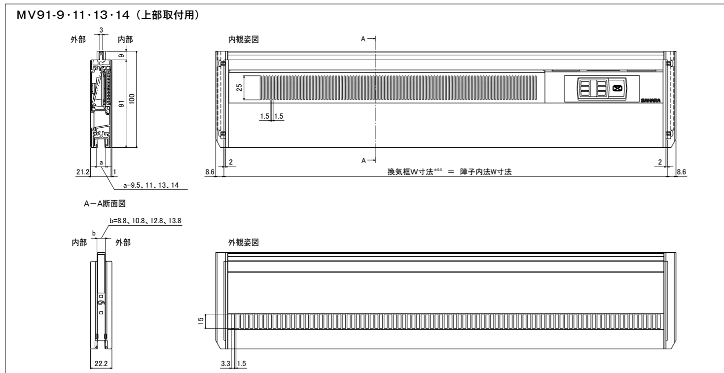
商品図
